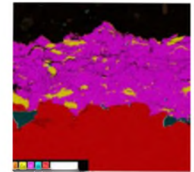
Структура покрытий на примере состава Ni-Cu (энергодисперсионный анализ)
