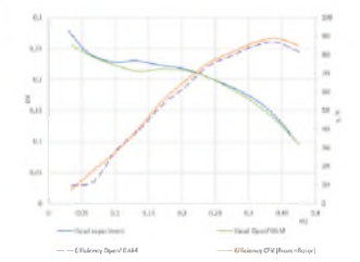
Рис. 5. Сравнение результатов численного моделирования с экспериментом
